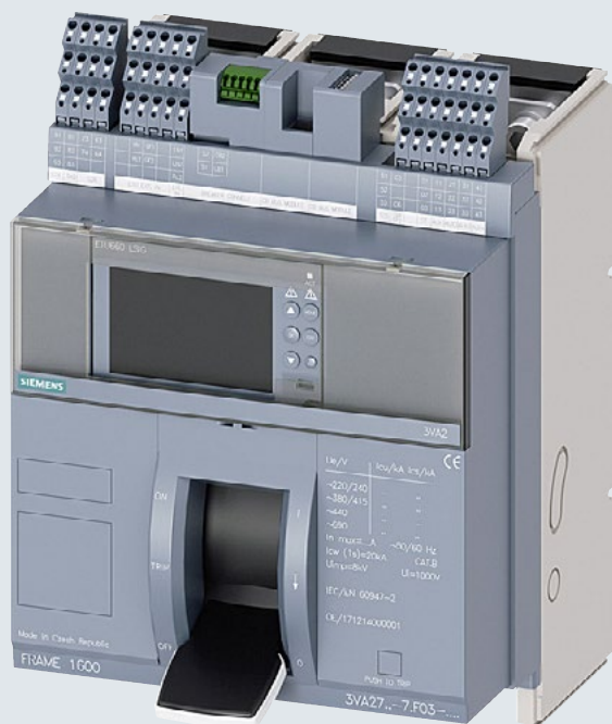
Выключатель в литом корпусе 3VA27
